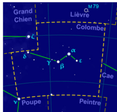
Carte du ciel, constellation de la Colombe
